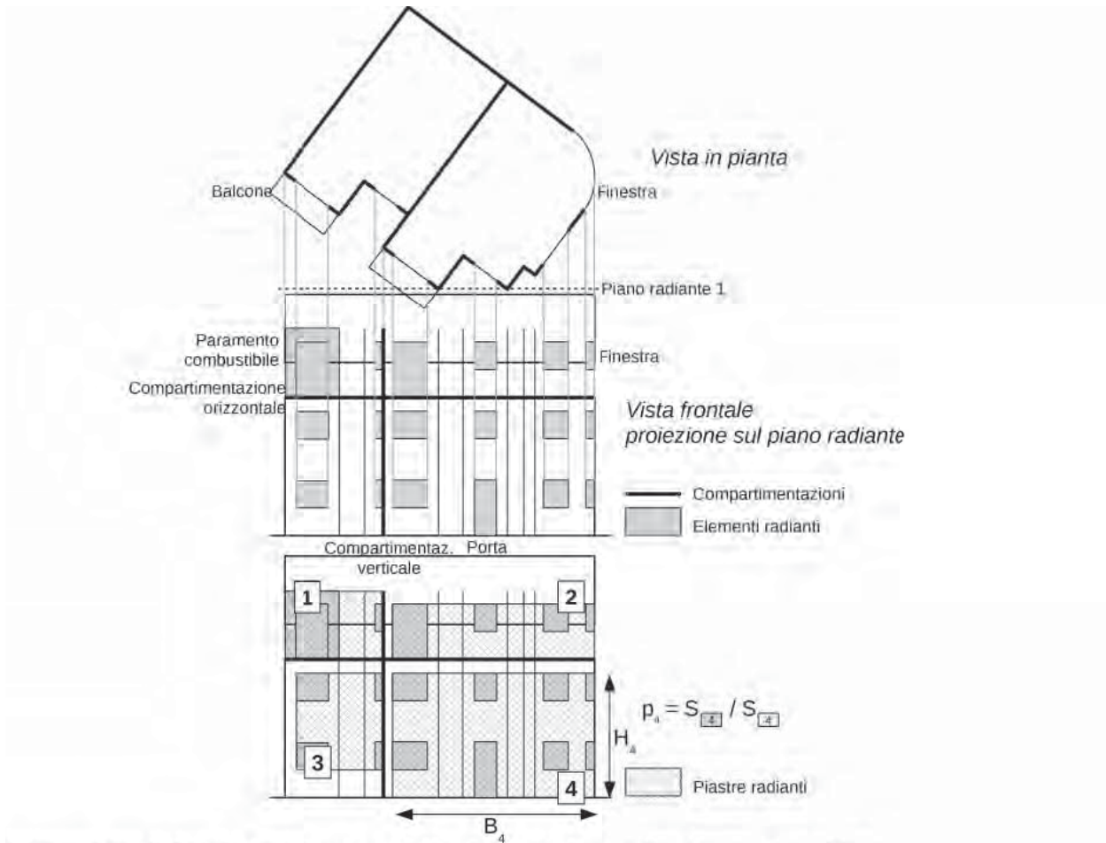
Illustrazione S.3-3: Determinazione delle piastre radianti, vista in pianta e frontale
