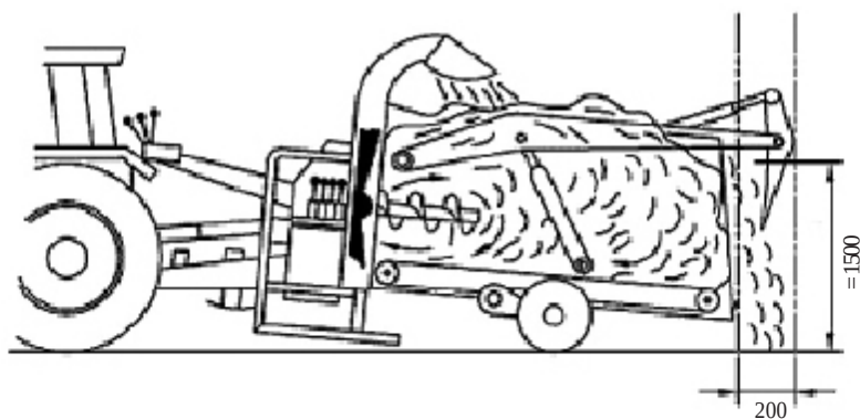
Figura 2. Aree di lavoro per la verifica della visibilità diretta per le macchine trainate. Dimensioni in mm
