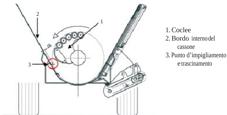
Figura 5. Esempio di punto in cui può verificarsi l'impigliamento e il trascinamento per il contatto con il dispositivo di miscelazione (coclee)
