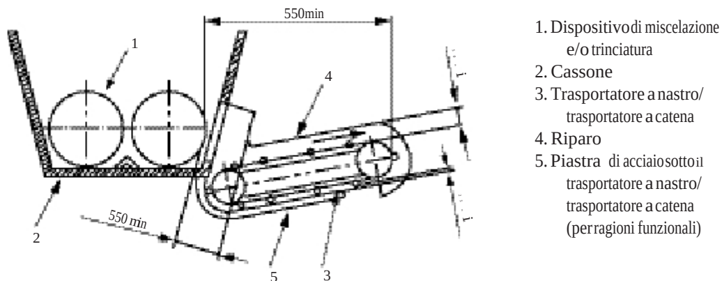
Figura 7. Protezione contro l'accesso diretto all'apertura di scarico quando è posizionata lateralmente (caso di un trasportatore con catena di acciaio). Dimensioni in mm
