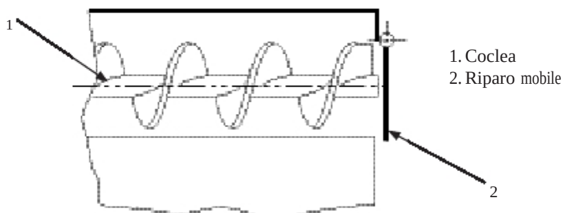
Figura 8. Riparo mobile a chiusura automatica per la protezione della coclea
